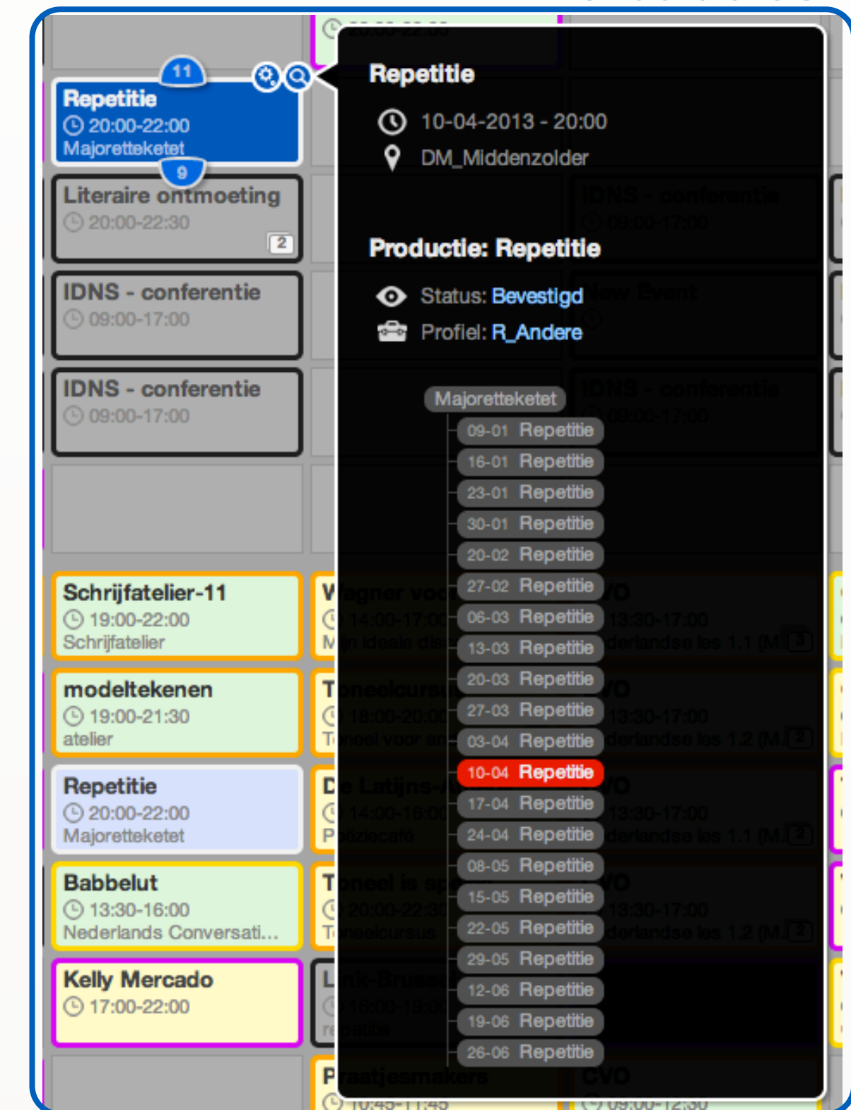
info bubbles
